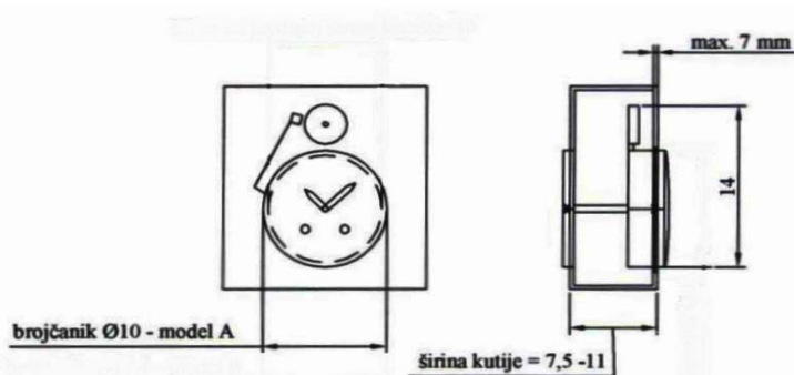
SKICA ZA MONTAŽU MEHANIZMA SA BROJČANIKOM MODEL A
